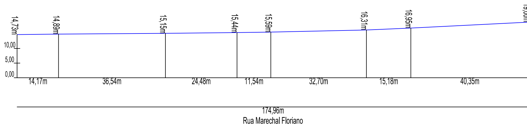
Perfil Longitudinal do trecho Escala: 1/750
