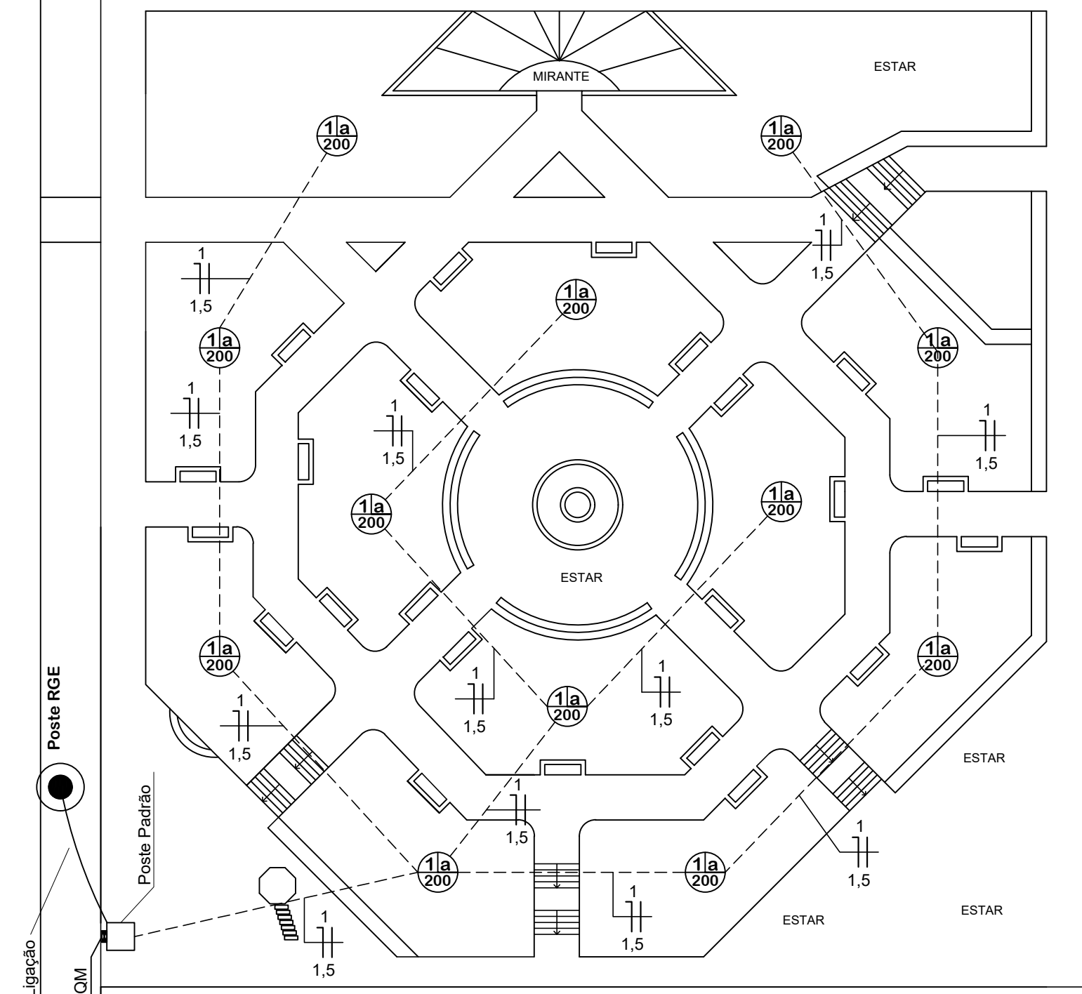
Planta Baixa Elétrica : PRAÇA Escala : 1 : 250
