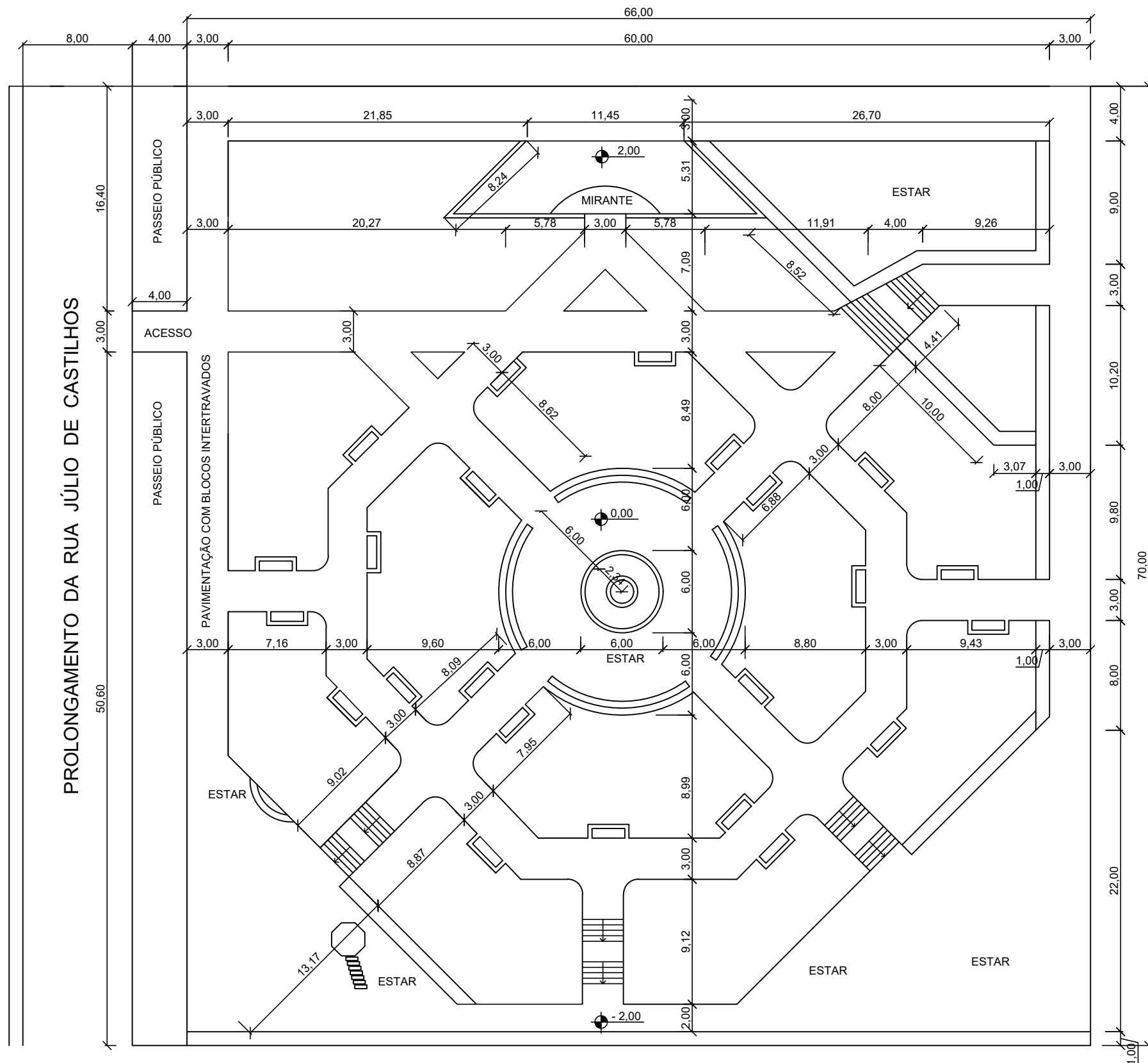
Planta Baixa : PRAÇA ÁREA CONSTRUÍDA DA PRAÇA : ....4.690,00 m 2 Escala : 1 : 250
