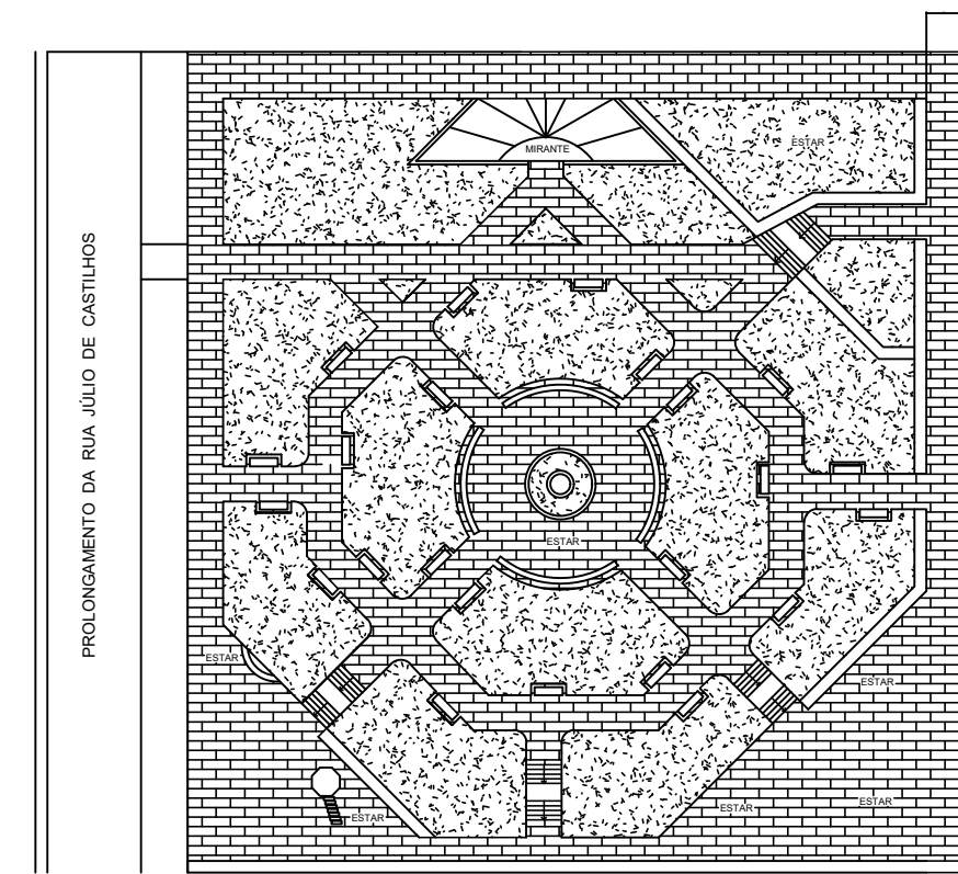
Planta Baixa : PRAÇA ÁREA A PAVIMENTAR : 2.150,00 m 2 Escala : 1 : 500 Pavimentação com blocos intertravados de concreto
