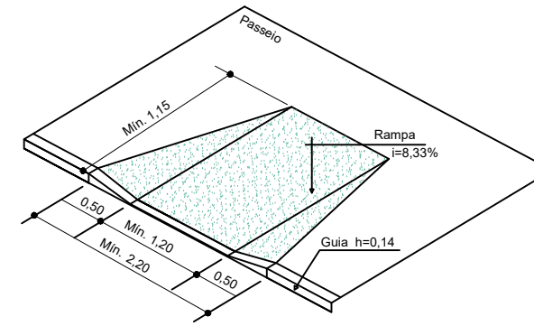
DETALHAMENTO RAMPA DE ACESSIBILIDADE S/escala
